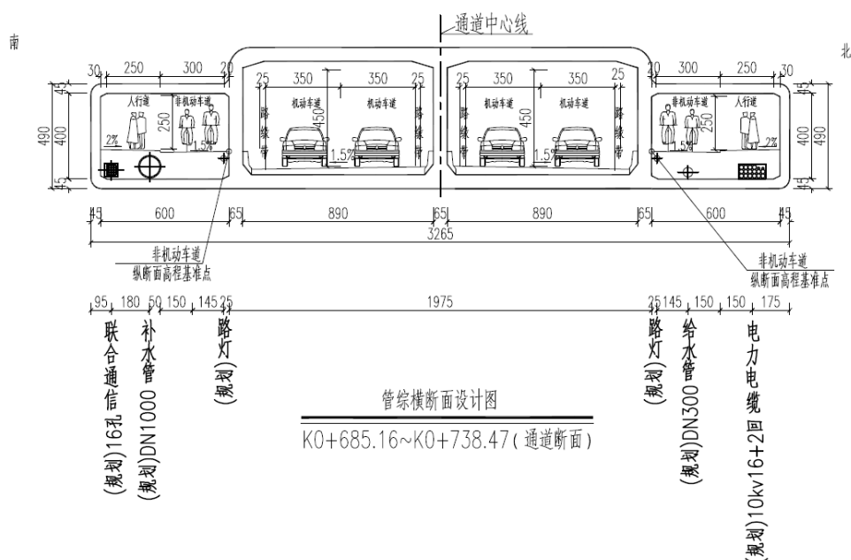
图1-9 桥涵工程管线综合标准横断面图
