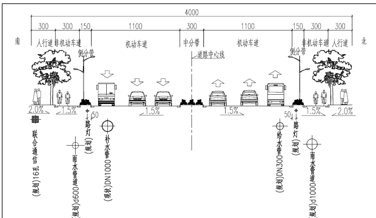
图1-8 交叉口管线综合标准横断面图
