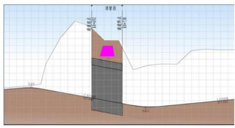
图 1-5 本项目桥涵纵断面图
