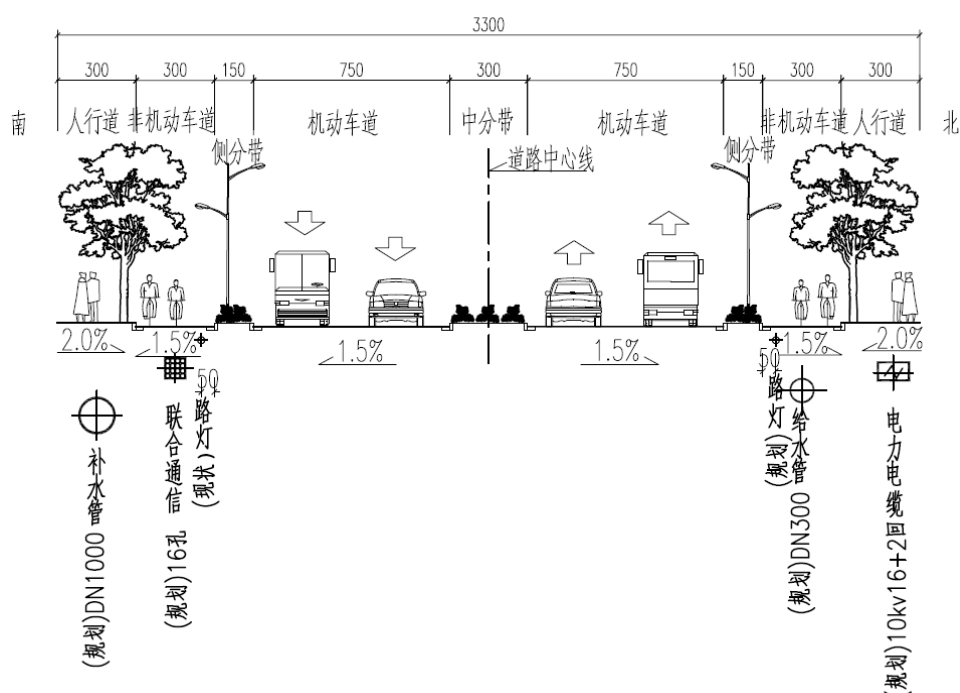
图1-7 道路管线综合标准横断面图
