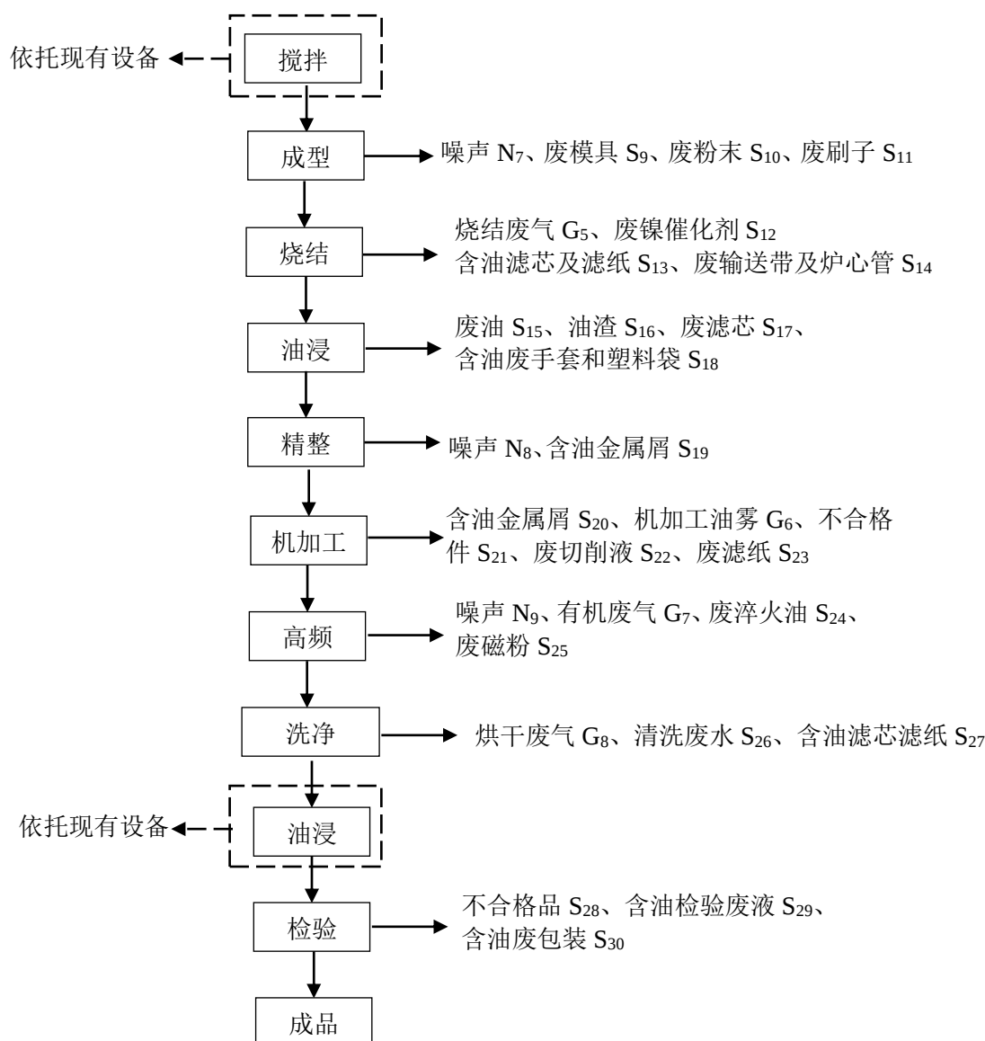
图 3.5-1 验收项目工艺流程及产污环节图
