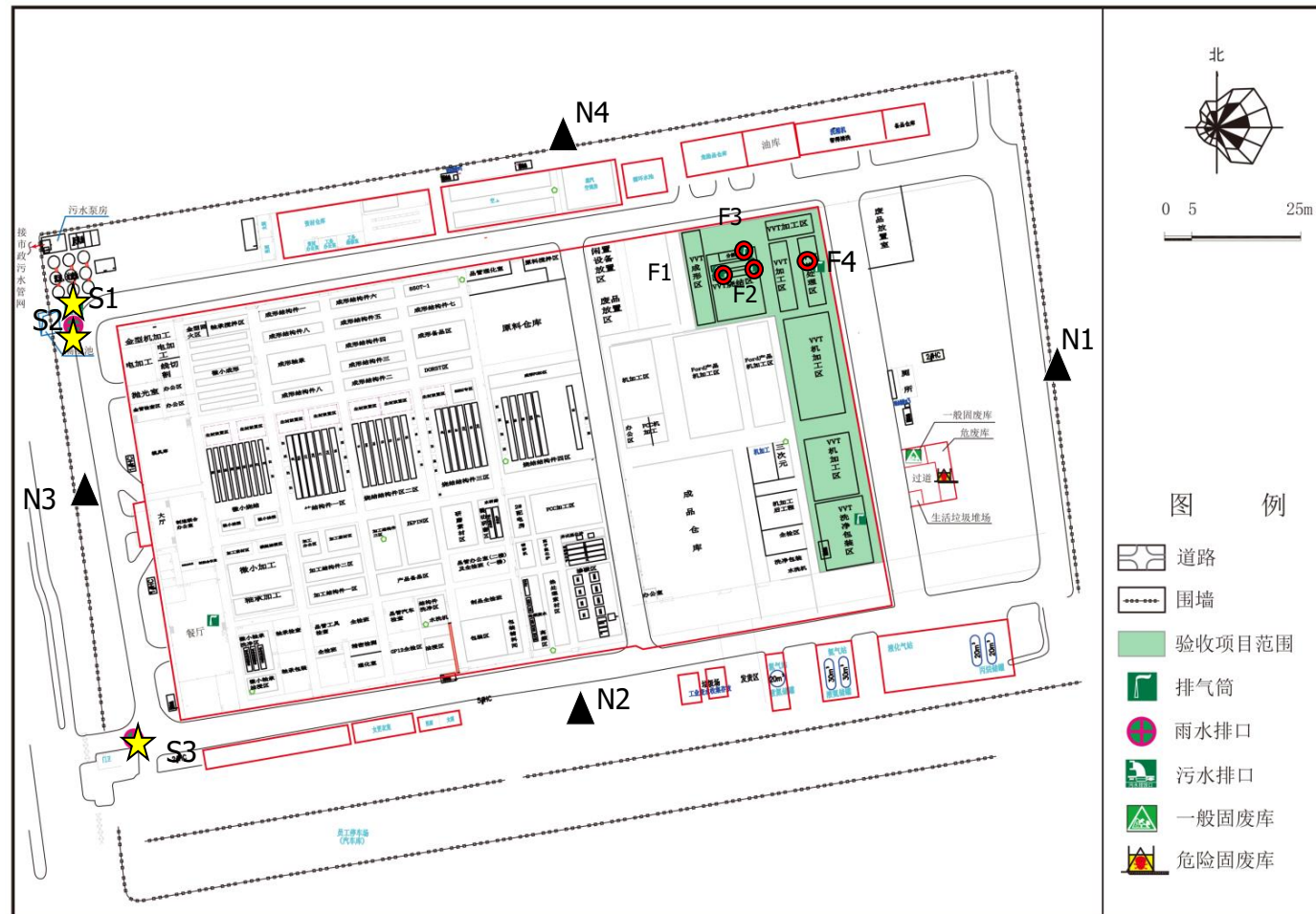
图 7.1-1 污染物监测点位示意图
