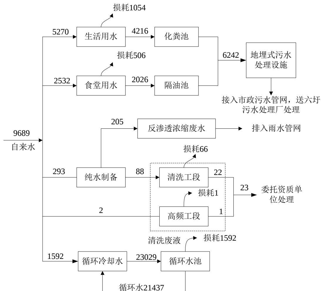
图 3.4-1 验收项目水平衡图
