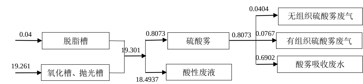
图 3.6-3 建设项目硫酸平衡图（单位：t/a）
