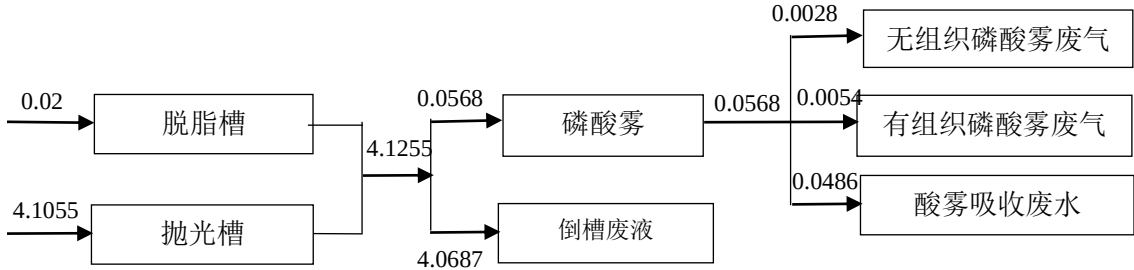
图 3.6-4 建设项目磷酸平衡图（单位：t/a）
