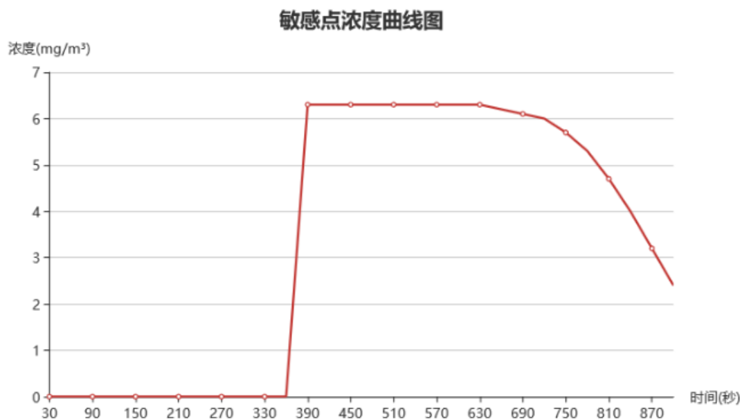
图 5.2.8-4 居民点 2 有毒有害物质浓度随时间变化情况
