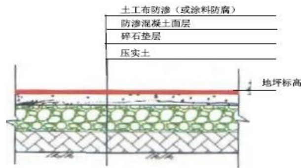
图 6.5-1 重点防渗区地面防渗结构图
