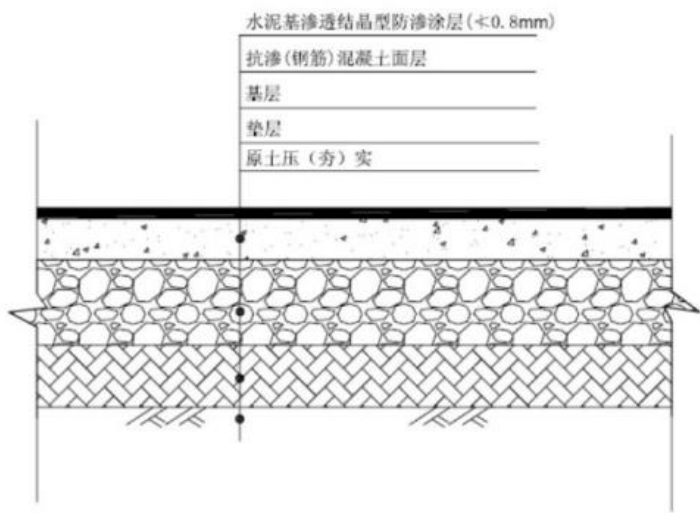
图 7.5-2 地坪重点防渗区域防渗结构
