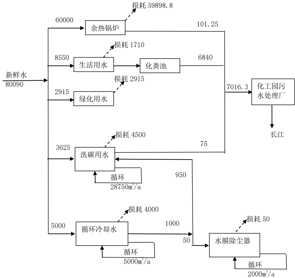
3.4-1 现有项目水、汽平衡图 单位t/a
