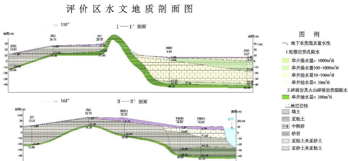
图 5.1-4 评价区水文地质剖面图
