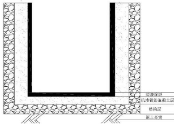
图 7.5-3 水池防渗结构
