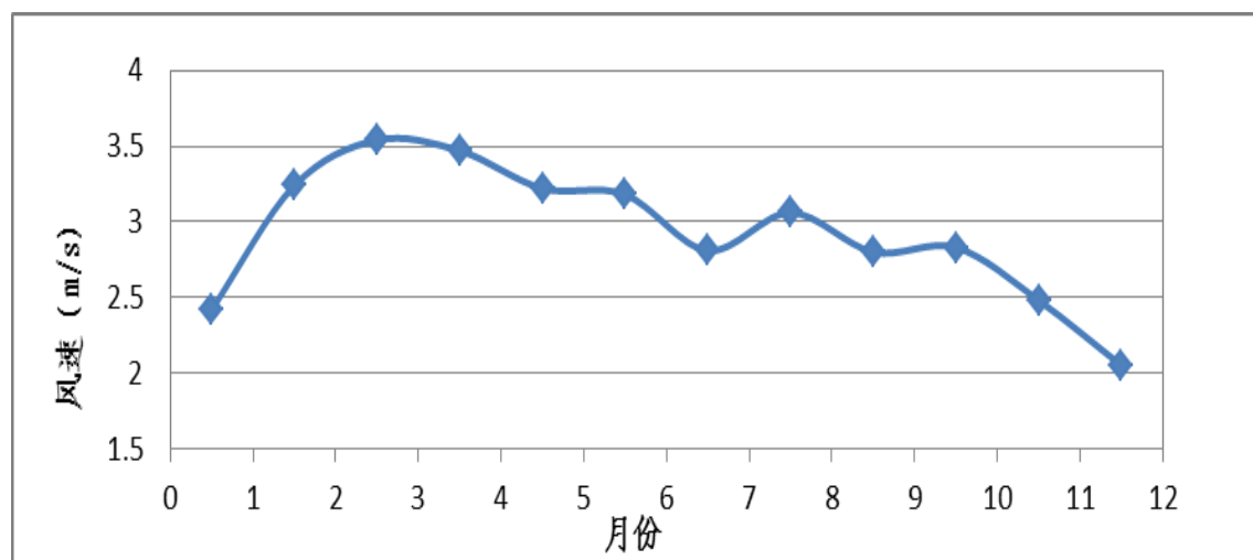
图 6.1-2 年平均风速的月变化图
