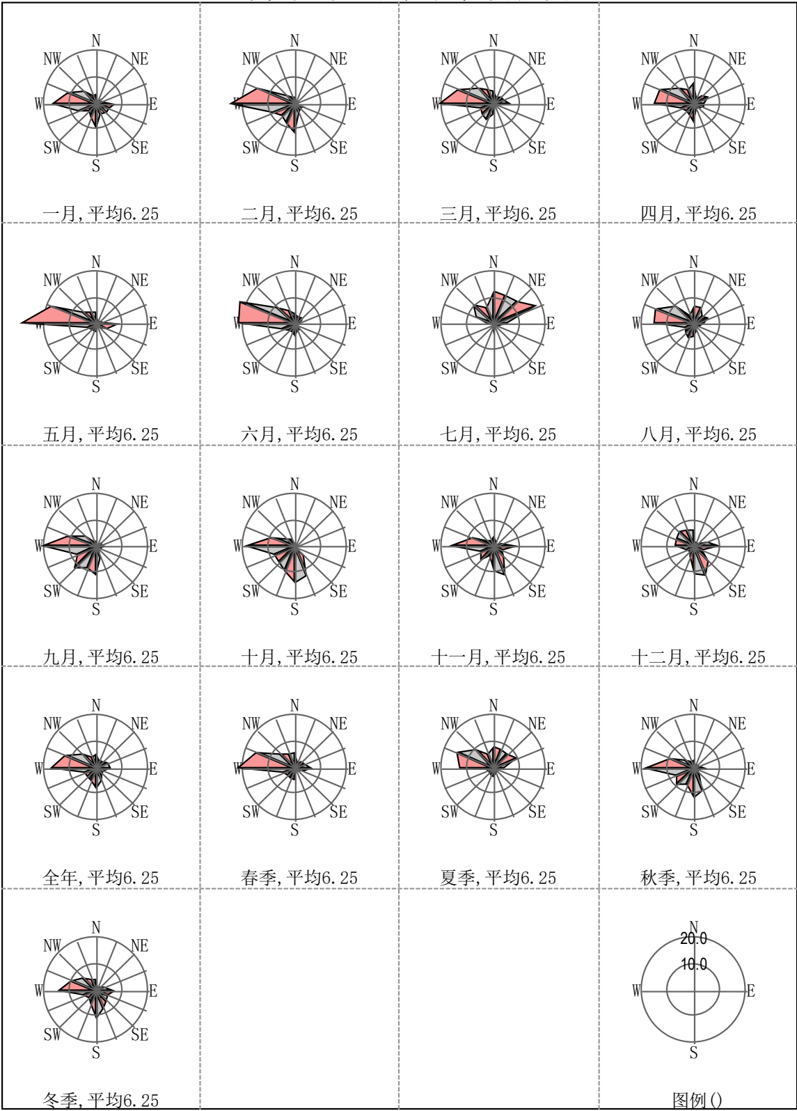
图 6.1-6 污染系数图
