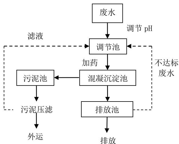
图 4 废水预处理工艺流程图
