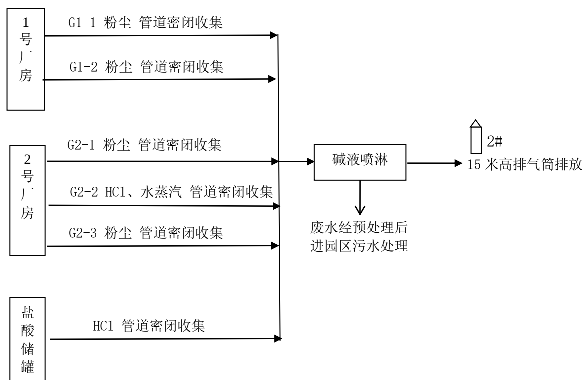
图 7.1-1 建设项目废气收集处理流程图
