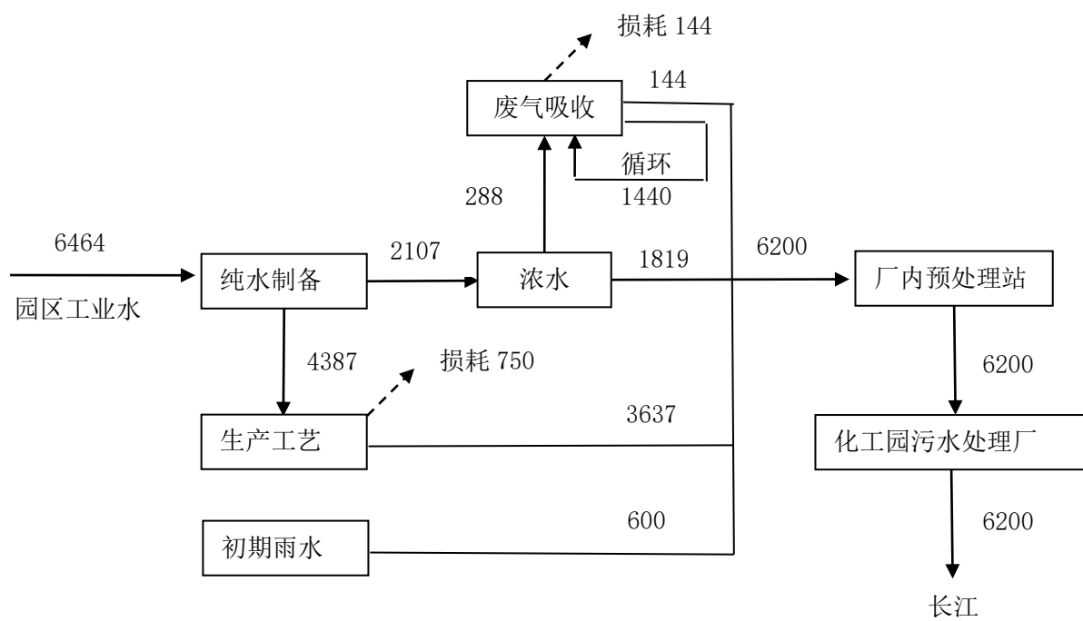
图 4.5-1 建设项目用水平衡图（单位：t/a）
