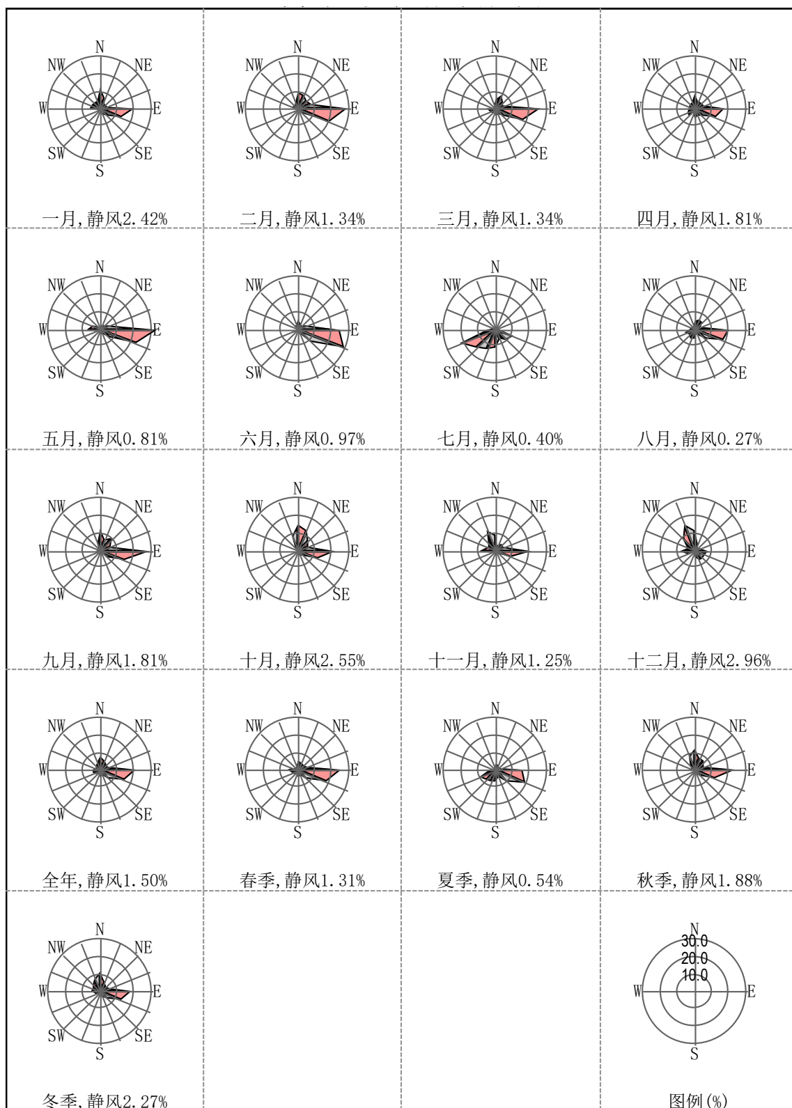
图 6.1-4 风向玫瑰图
