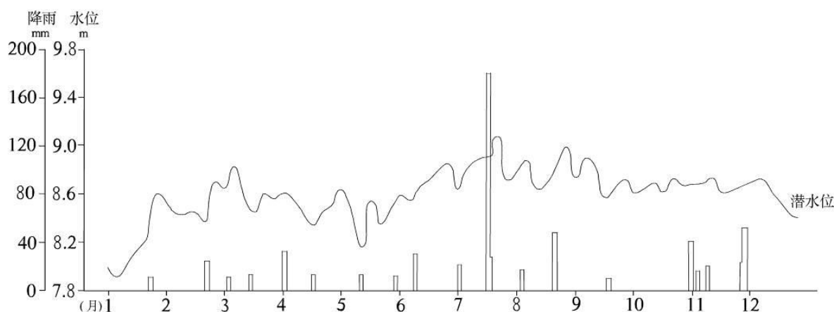
图 5.1-5 潜水位与降水关系图
