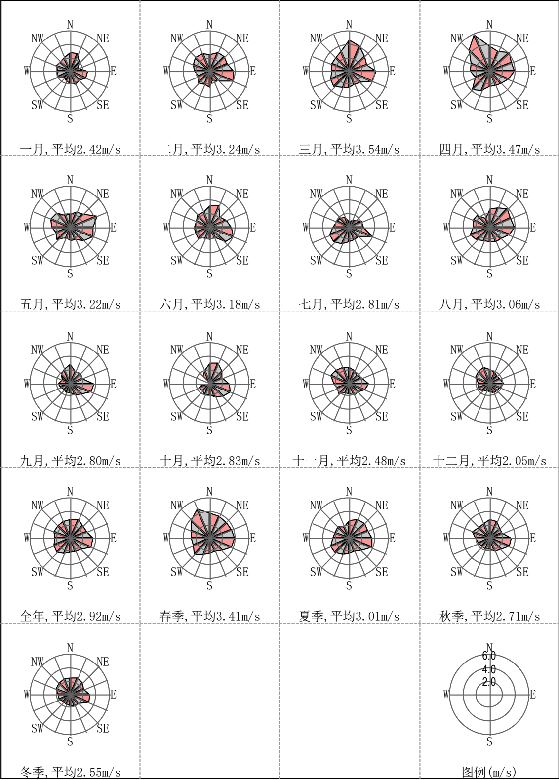
图 6.1-5 风速玫瑰图
