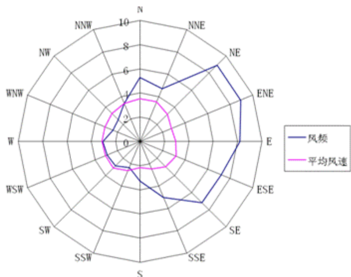
图 6.1-7 南京地区 1978-2013 年统计气象资料风玫瑰图
