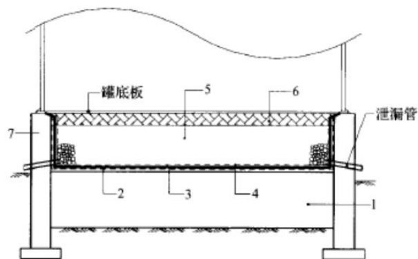
1-原土夯实；2-膜下保护层；3-HDPE 土工膜（2mm）； 4-膜上保护层；5-砂垫层；6-沥青层；7-环墙基础。
